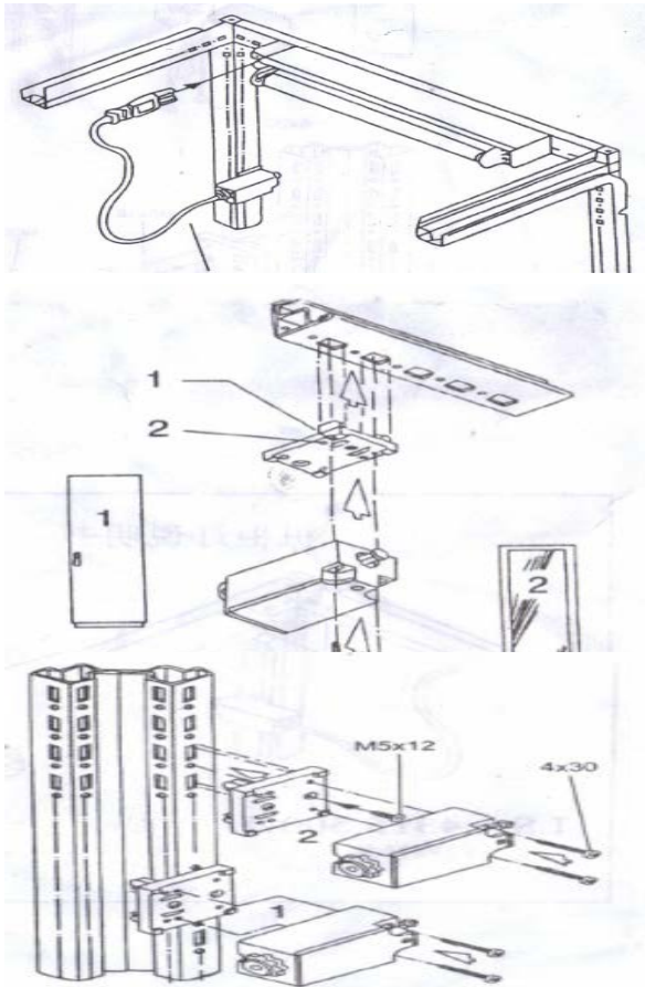
门控开关安装使用示意图：
